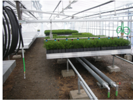
苗木を設置。下部2本のパイプは温水を循環させる加温設備、上部から吊り下げられた器材は温湿度を調節するミスト用ノズル。
