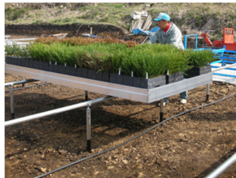
カートから屋外順化場所へのベンチ移動も一人で可能。少しの力で移動可能であり、全ての作業をベンチ上で立て行えるので、労働負荷が少なく、作業効率も向上する。
