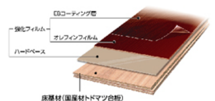
ベリッシュ シスト S-J 断面図
