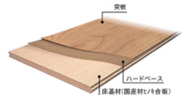
ベリッシュ カラーフロア TR-J 断面図
