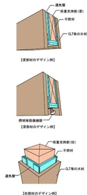
【柱部材のデザイン例】
