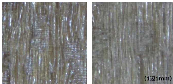
図3 宇宙曝露後木材試験体(ホオノキ)拡大写真 左:宇宙曝露試験体 右:宇宙未曝露試験体
